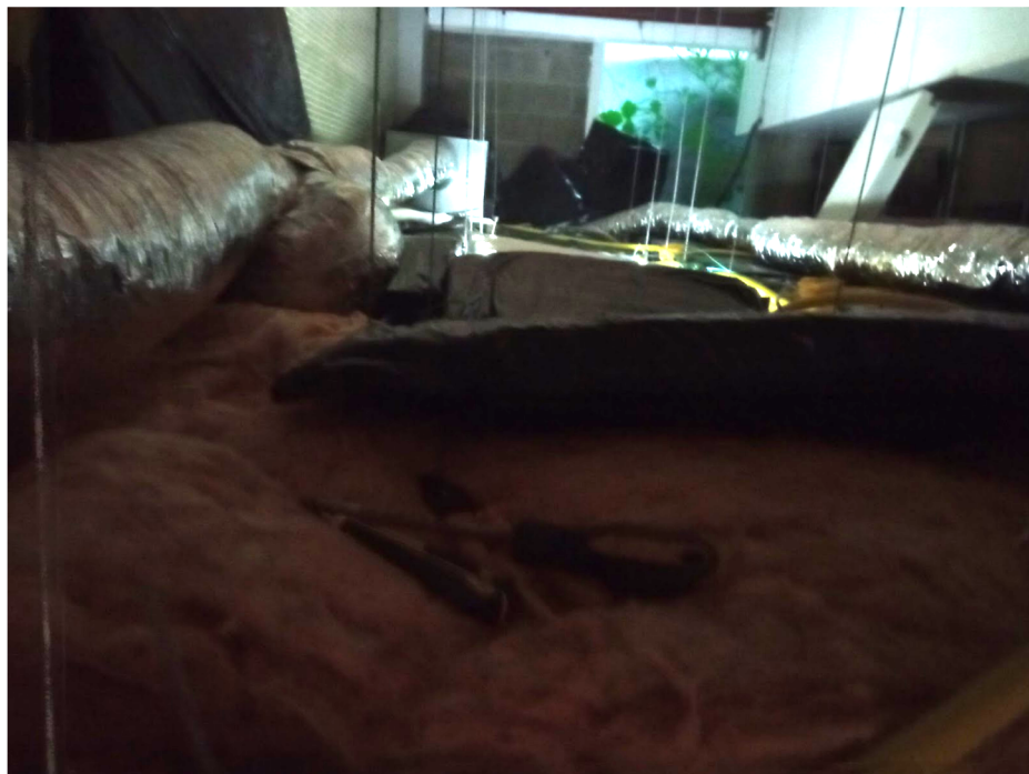
Figura 6 - Instalação de lâ de rocha sobre teto de gesso, instalação de tubulações de ventilação/exaustão e instalação de caixa de ventilação.
