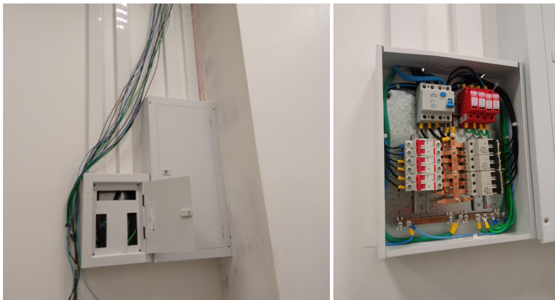
Figura 12 - Instalação de quadro de distribuição de energia elétrica e disjuntores.
