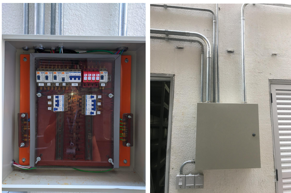
Foto 04 - Quadro de distribuição de energia.
